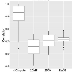
scm3C-seq
