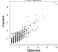
HiImpute
