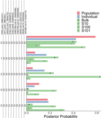
Fig 19: Posterior Distribution of Patient 1
