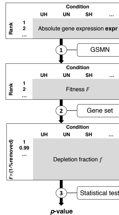
Fig. 4. metaboGSE algorithm.
