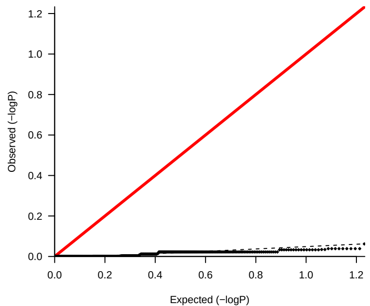
lambda 0.059
