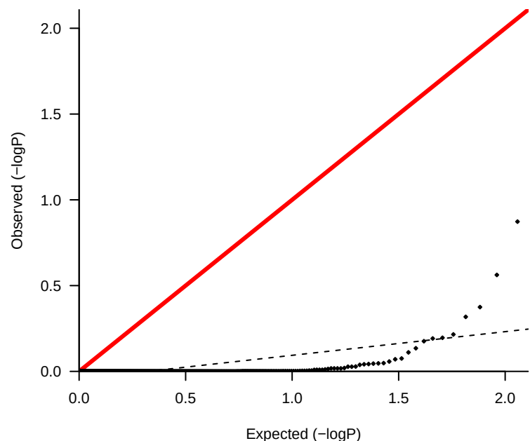
lambda 0.138
