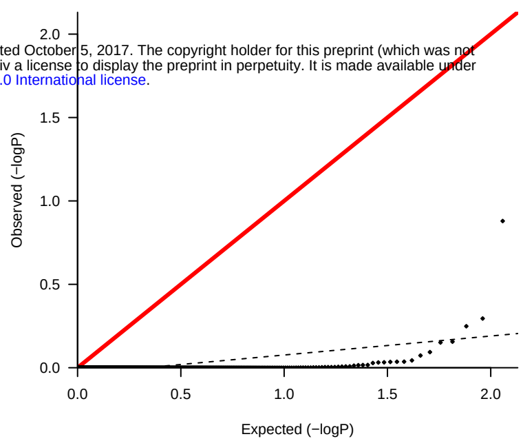
lambda 0.114
