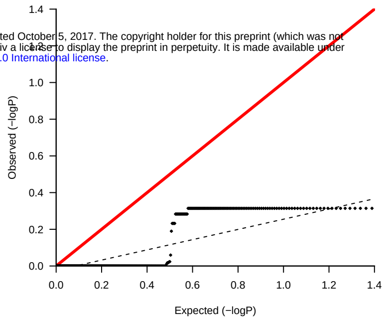
lambda 0.279
