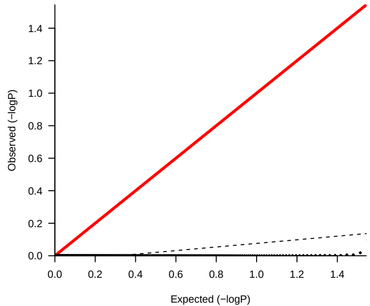
lambda 0.111
