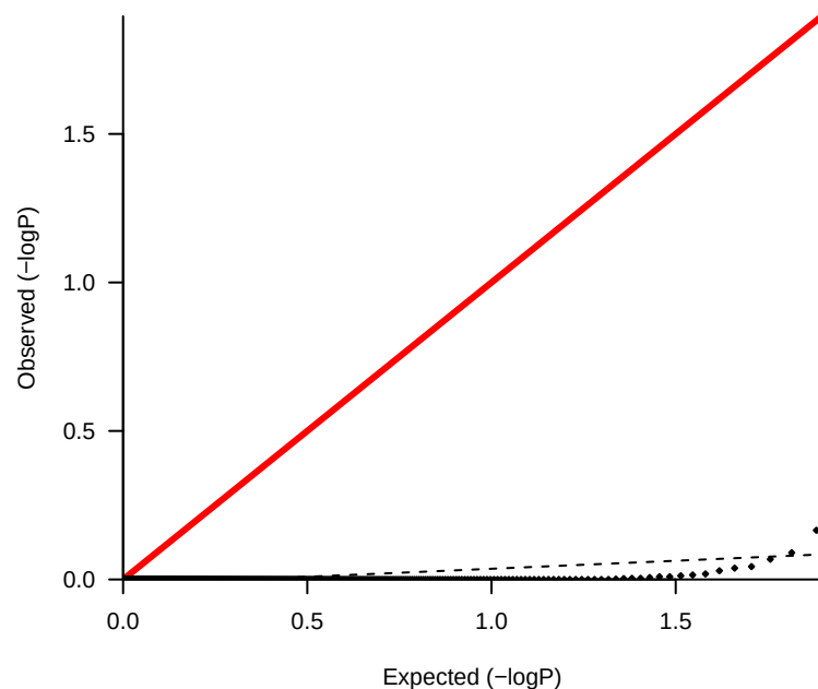
lambda 0.054
