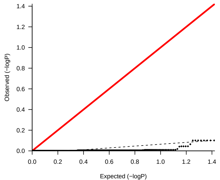
lambda 0.089
