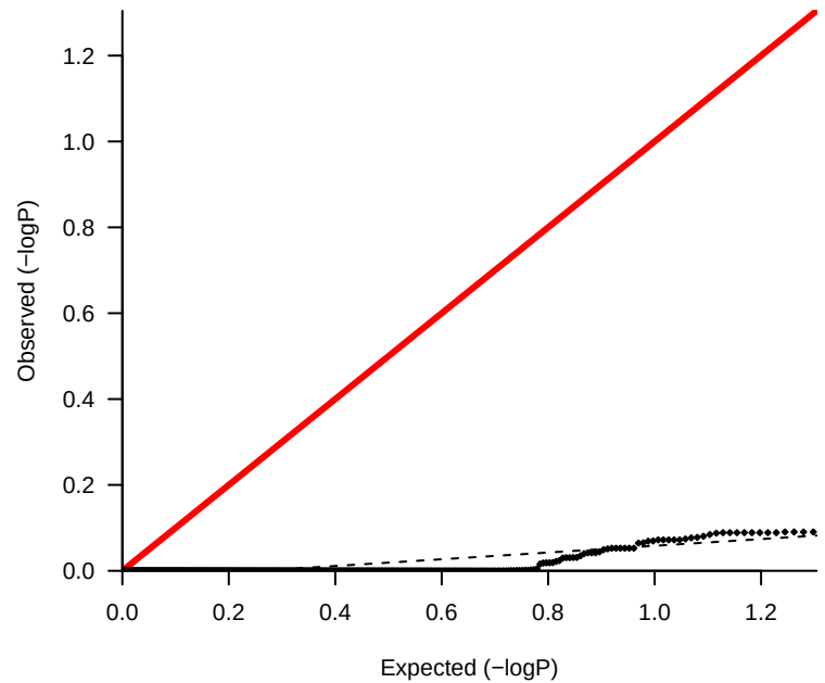
lambda 0.078
