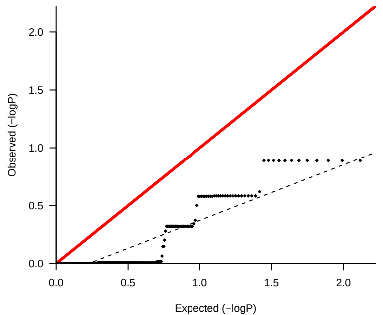
lambda 0.481
