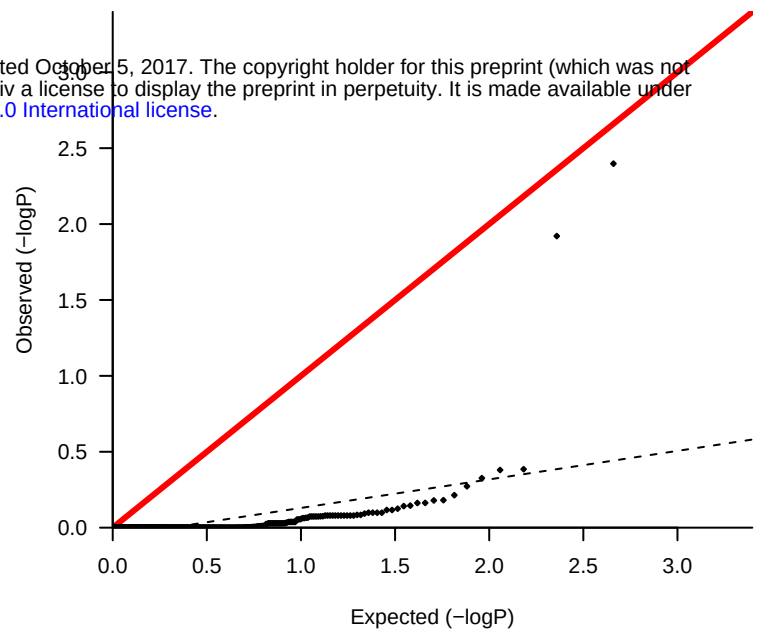
lambda 0.188
