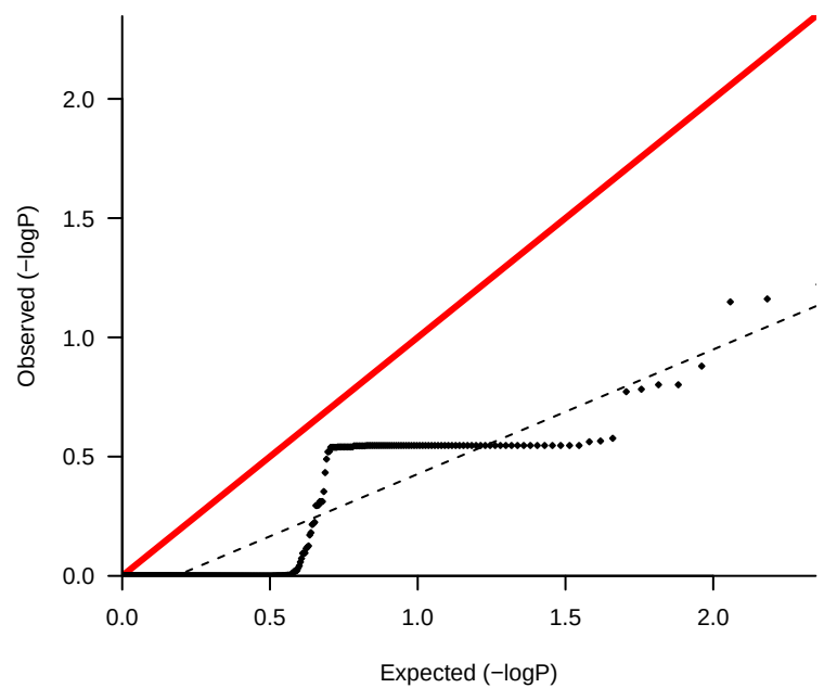
lambda 0.522
